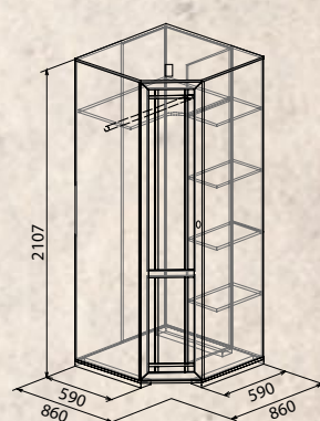
Sherlock 10 (гостиная) Шкаф угловой + фасад Стандарт
