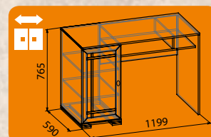
Sherlock 115 Стол письменный
