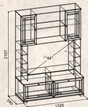
Sherlock 1 Шкаф МЦН
