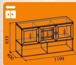
Sherlock 4 (гостиная) Шкаф навесной
