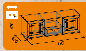
Sherlock 3 Тумба ТВ
