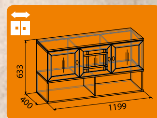
Sherlock 4 (гостиная) Шкаф навесной
