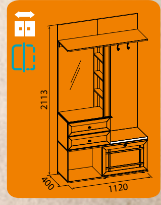
Sherlock 70 Шкаф МЦН
