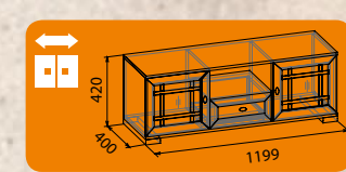
Sherlock 3 Тумба ТВ
