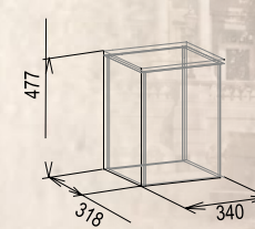
MONTPELLIER (спальня) Банкетка 1
