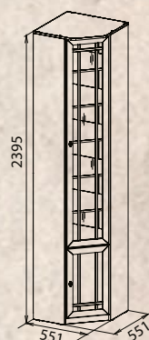
Sherlock 33 Шкаф для книг
