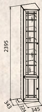
Sherlock 34 Шкаф для книг
