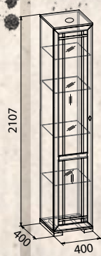
Sherlock 13 Шкаф для посуды
