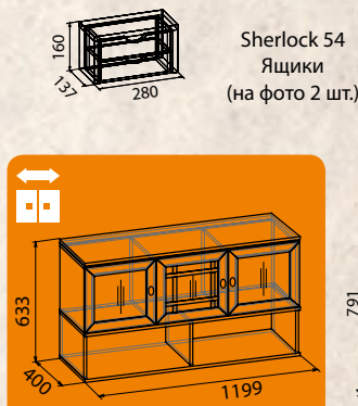
Sherlock 4 (гостинная) Шкаф навесной
